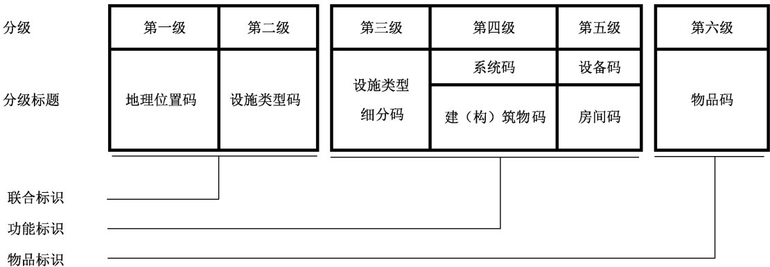
图 1 标识结构
